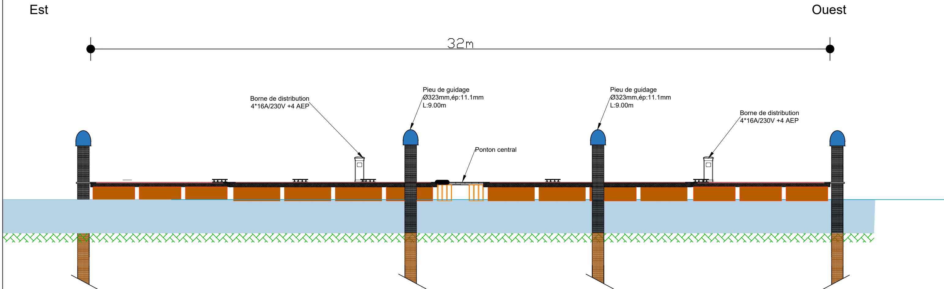
Coupe BB dans axe ponton d'extrémité- Echelle: 1/100
