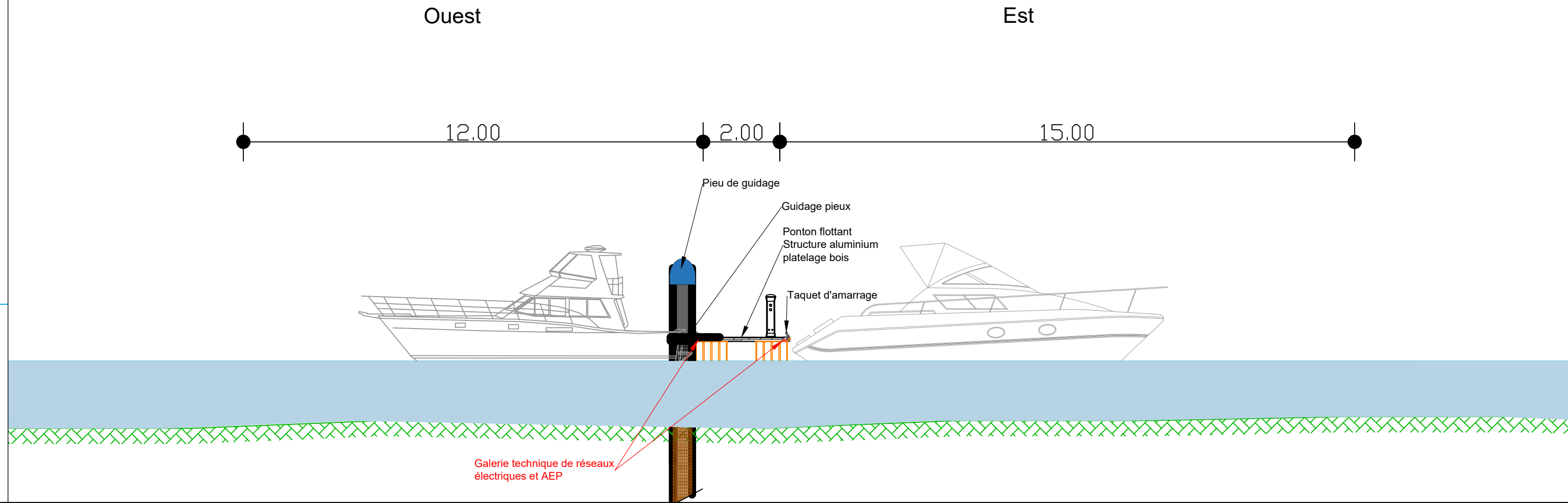
Coupe CC - Echelle: 1/200
