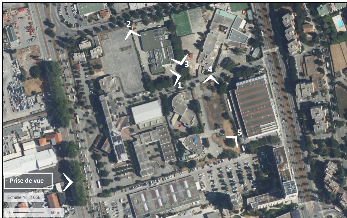
Localisation des prises de vue sur la zone d'étude (source : Copernicus)
