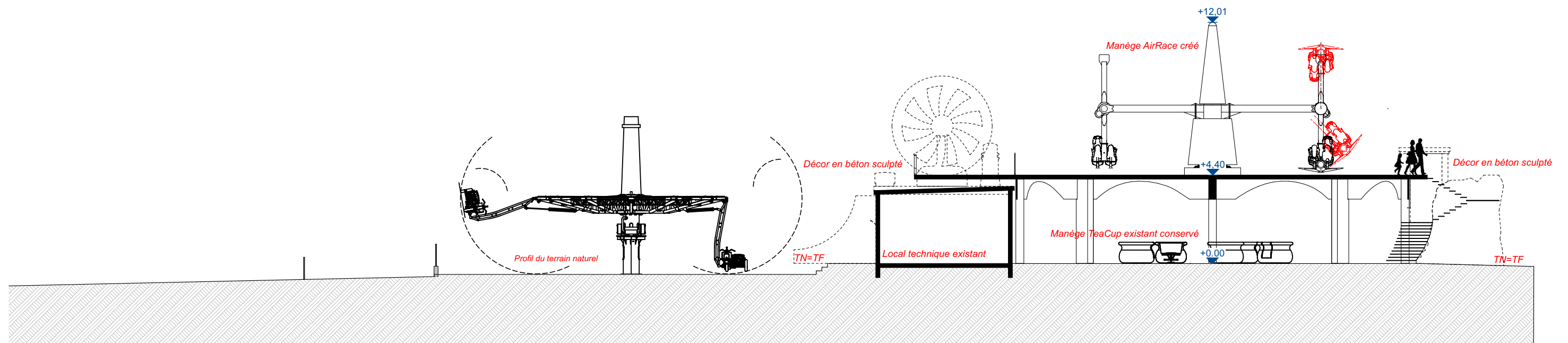
PC3 - Coupe Transversale - Projet -
