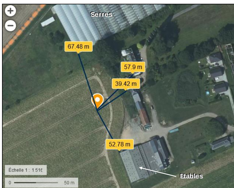
Situation du forage projeté par Madame Pauline LEMARCHAND à QUINCAMPOIX (76) sur photographies aériennes de l'IGN (Extrait de : geoportail.gouv.fr )
