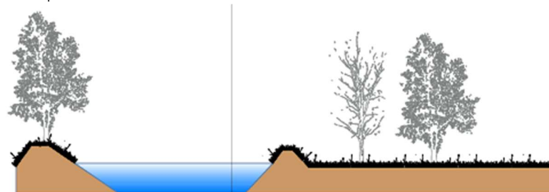
Coupe du bassin de rétention
