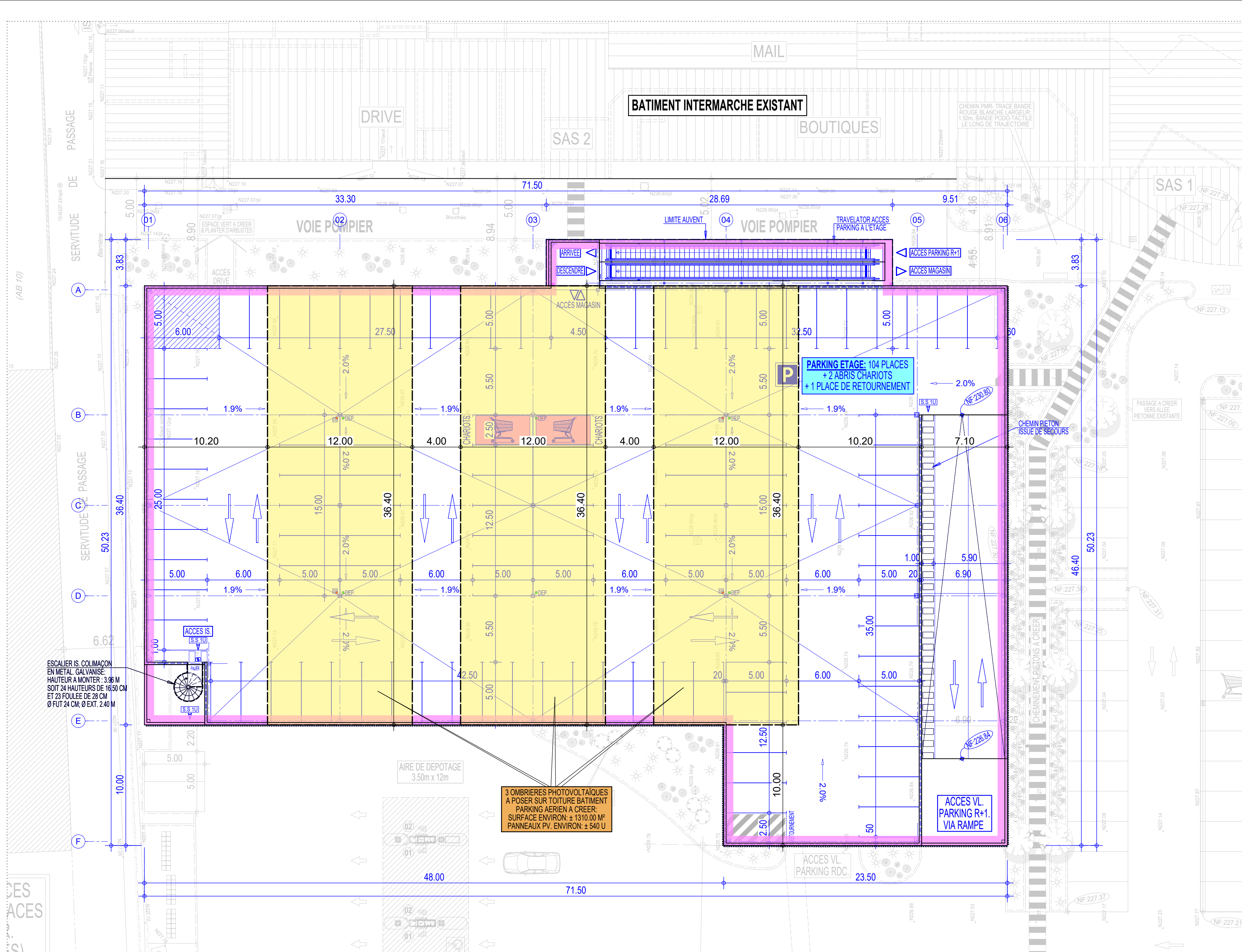
PLAN PARKING ETAGE & OMBRIERES - ECHELLE: 1/200
