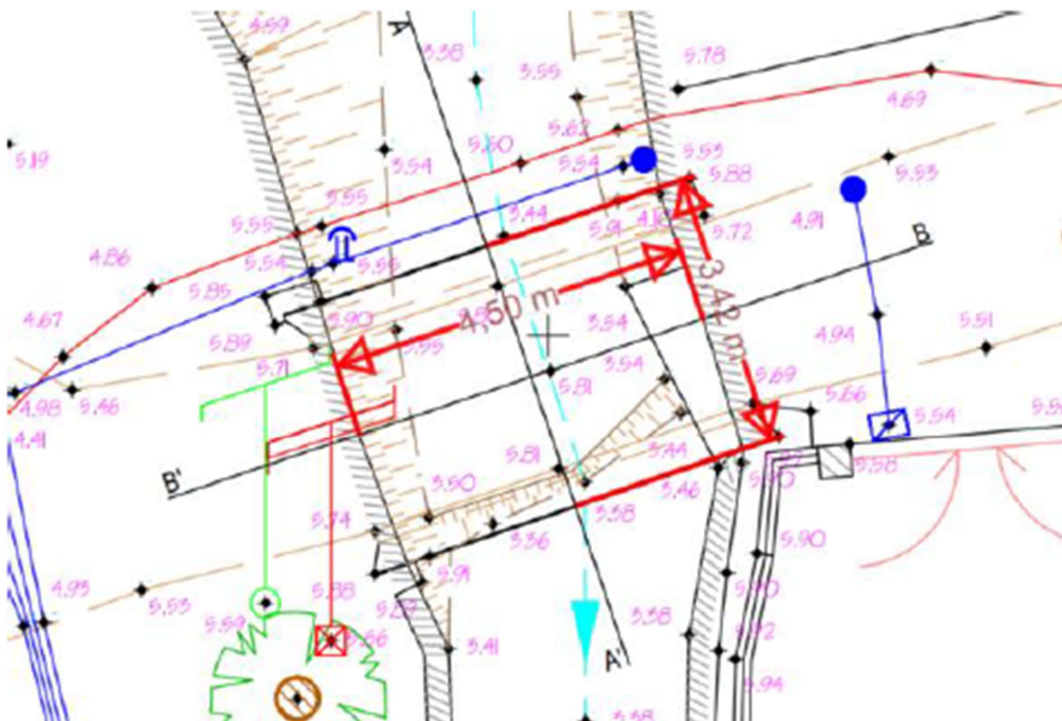
Vue en plan de l'ouvrage existant
