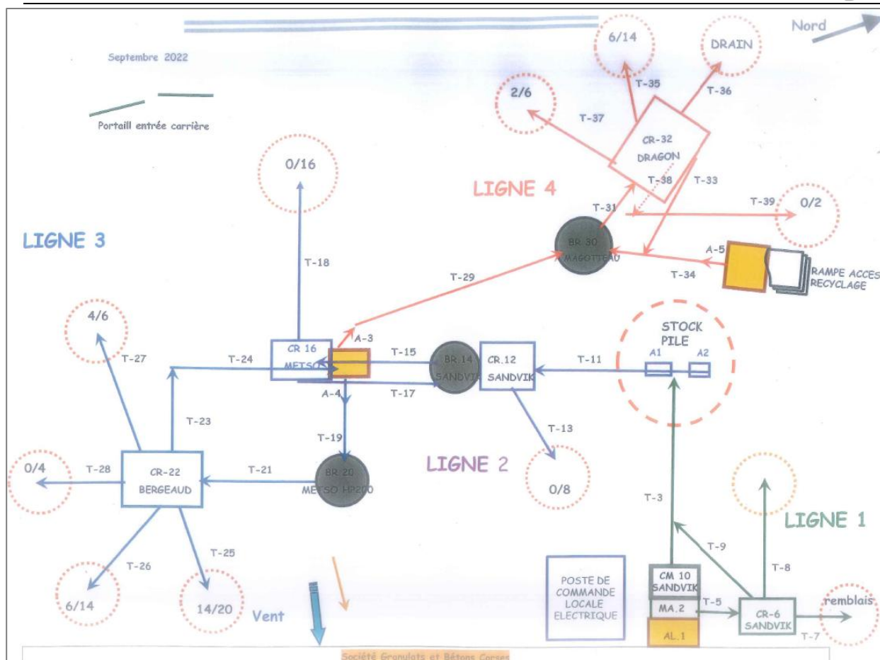
Figure 1. Synoptique schématique de l'installation de concassage-criblage
