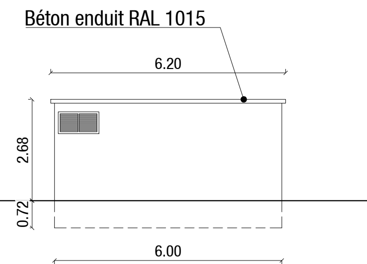
FAÇADE EST
