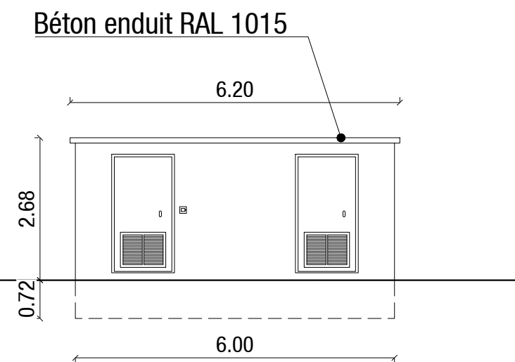
FAÇADE OUEST
