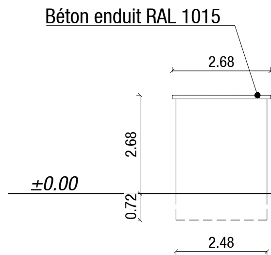
FAÇADE SUD
