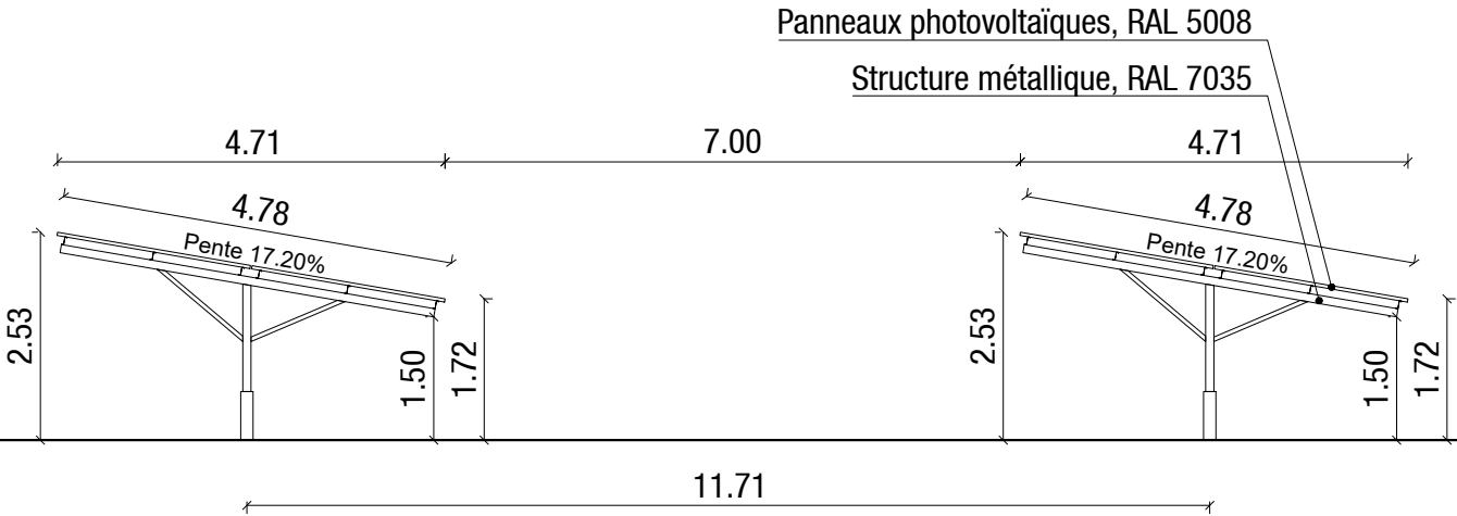
FAÇADE EST
