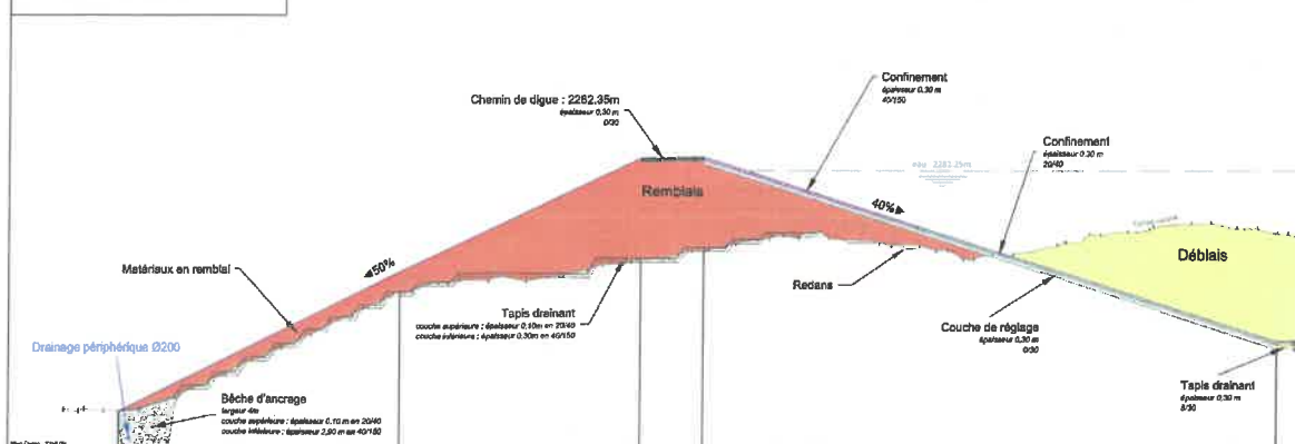
Coupe 2 : remblais échelle 1/250
