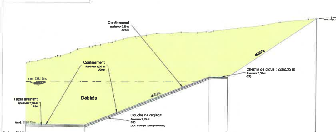
Coupe 1 : déblais échelle 1/250
