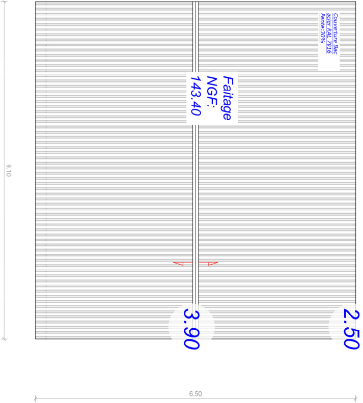
Toiture Bâtiment fouille pédagogique
