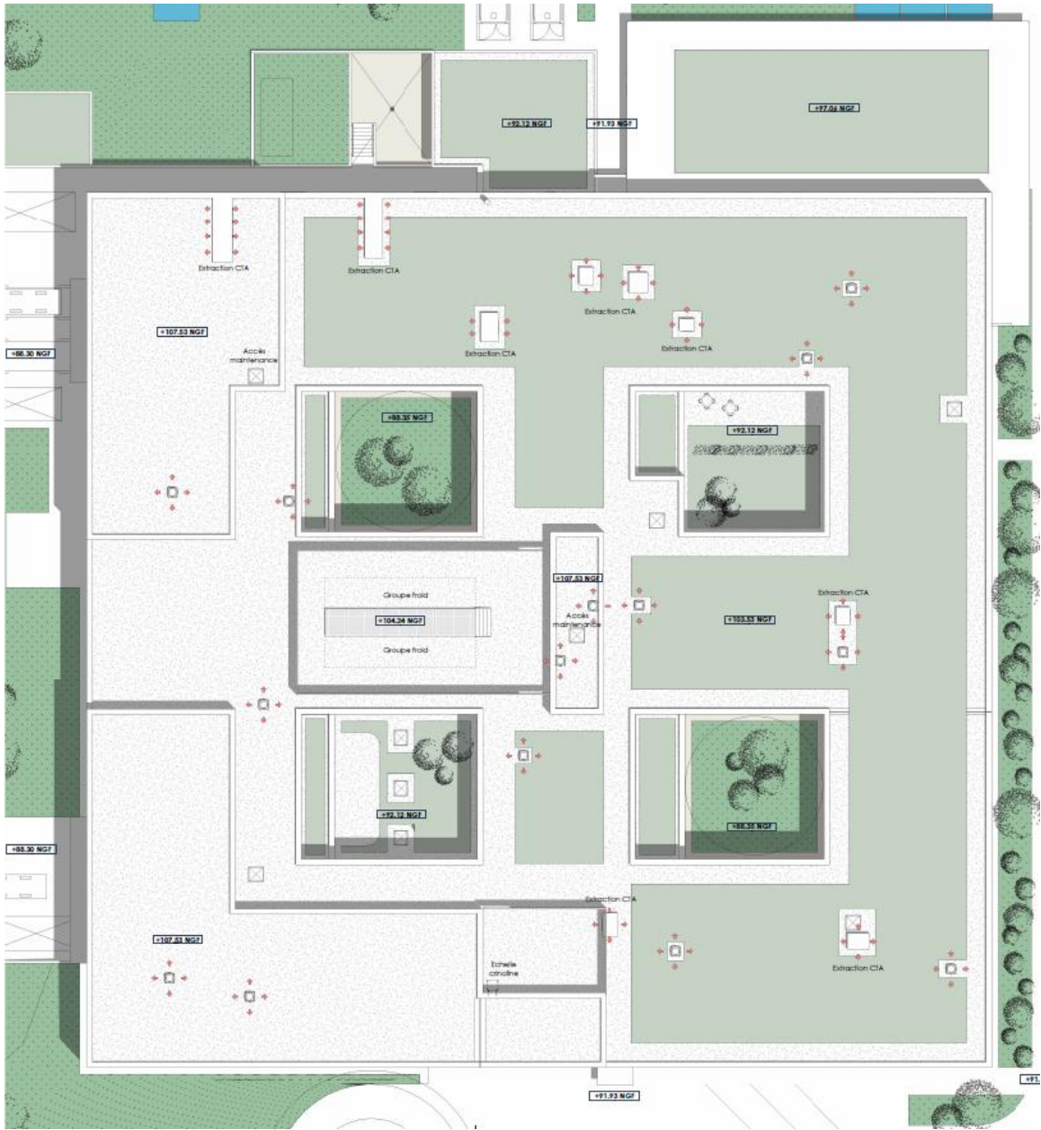
Plan de toiture (AFA + SANAE, 31/07/2026)
