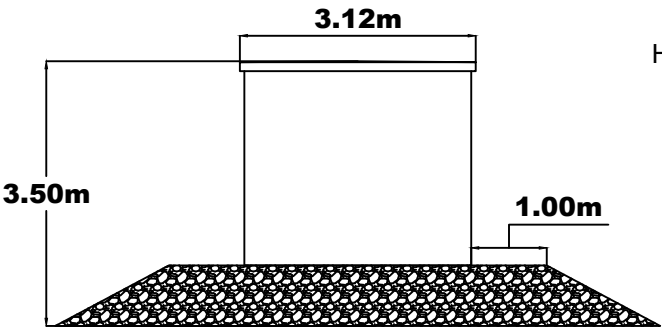
FACE GAUCHE
