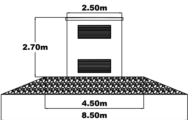
FACE DROITE
