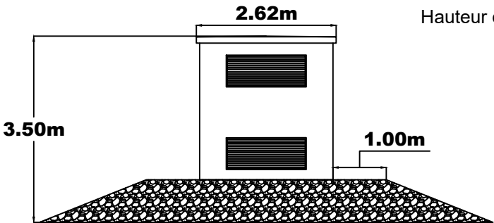
FACE GAUCHE
