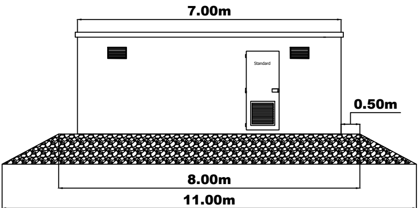
FACE ARRIERE
