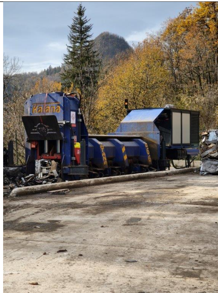
Photo n°6 : presse cisaille
