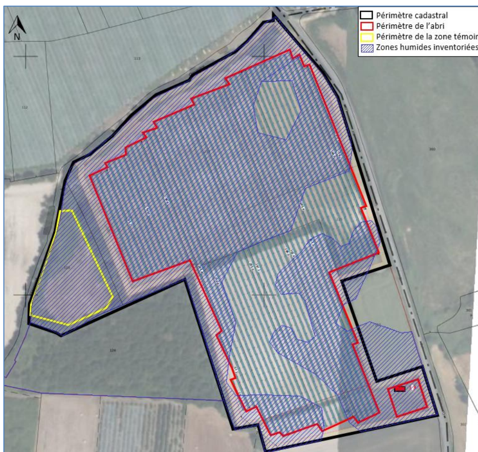
Figure 9 : Plan de masse du projet initial d'abri climatique sur une vue aérienne [Technique Solaire, 10/04/2024]
