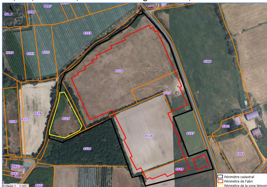
Figure 2 : Plan des emprises du projet d'abri climatique initial sur une vue aérienne au 1/ 2 000 ème [Géoportail]
