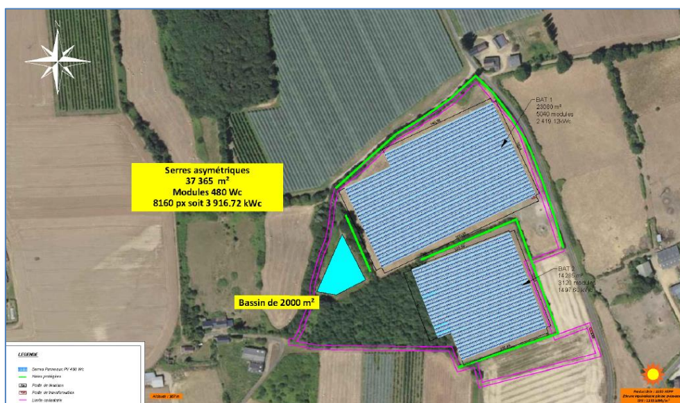
Figure 8 : Plan de masse du projet de serres photovoltaïques [Amarenco Construction, Octobre 2021]
