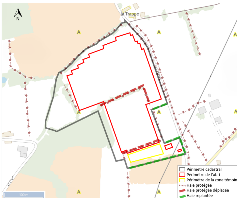
Figure 7 : Localisation du projet par rapport au PLU en vigueur et des haies protégées préservées, déplacées et replantées [Géoportail de l'urbanisme, Technique Solaire]
