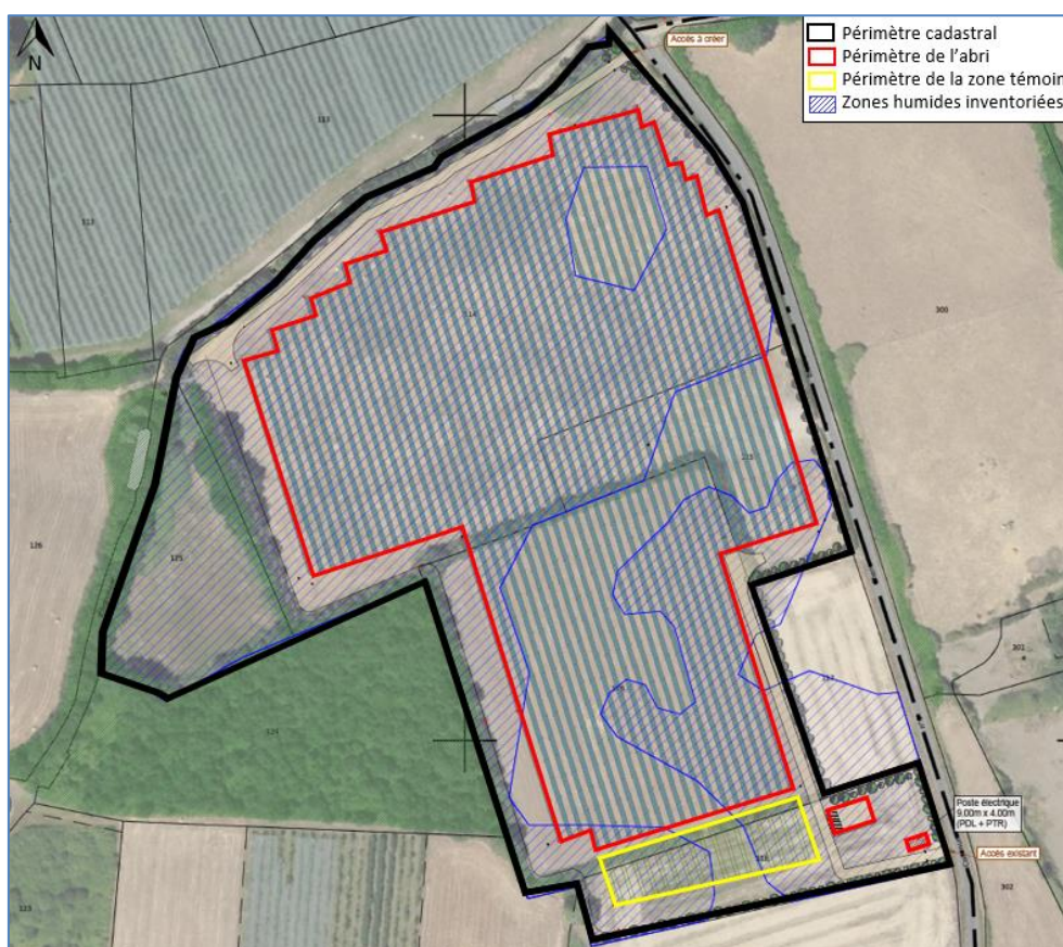
Figure 10 : Plan de masse du projet final d'abri climatique sur une vue aérienne [Technique Solaire, 20/02/2025]
