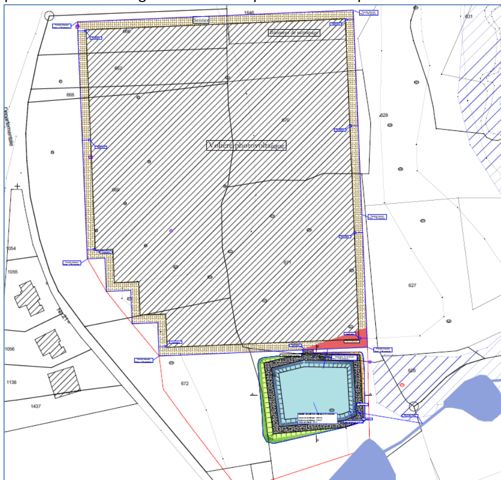
Figure 12 : Proposition de gestion des eaux pluviales sur le site du projet [AGGRA Concept, V2, 08/04/2025]
