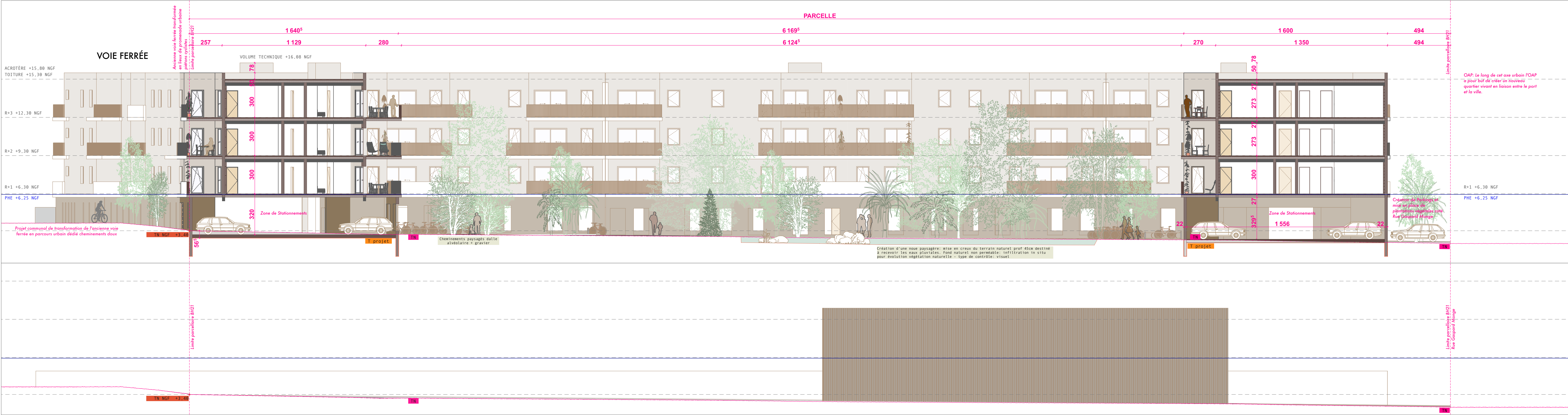
PC03 - COUPE A1 Ech. 1/150 - Sur l'ensemble de la parcelle et ses abords Bas - Coupe du profil terrain et ses constructions existants Haut - Coupe du profil, des constructions et des aménagements projetés
