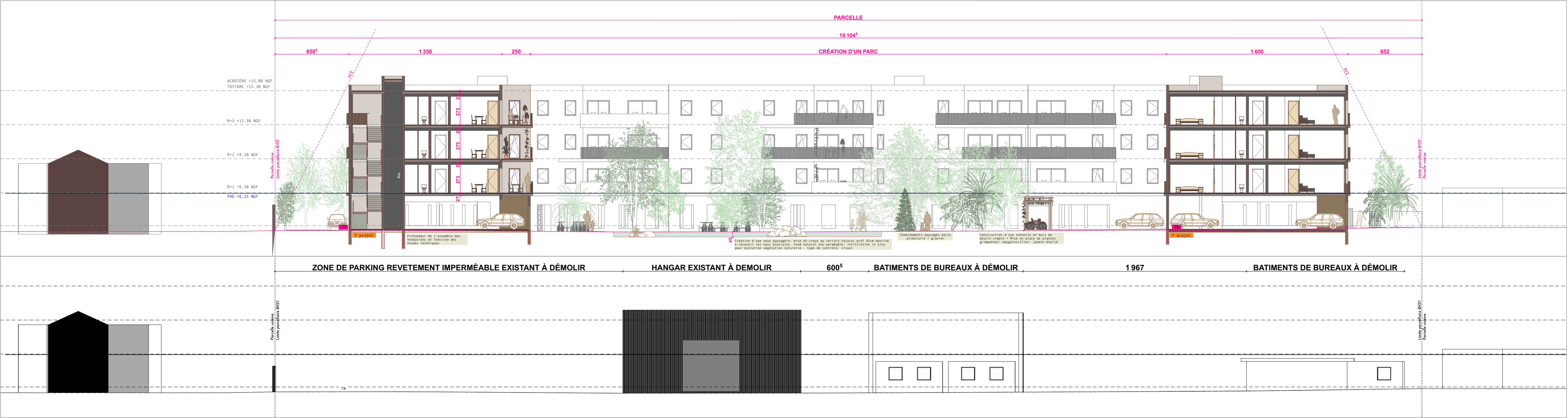
PC03 - COUPE B1 Ech. 1/200 Sur l'ensemble de la parcelle et ses abords
