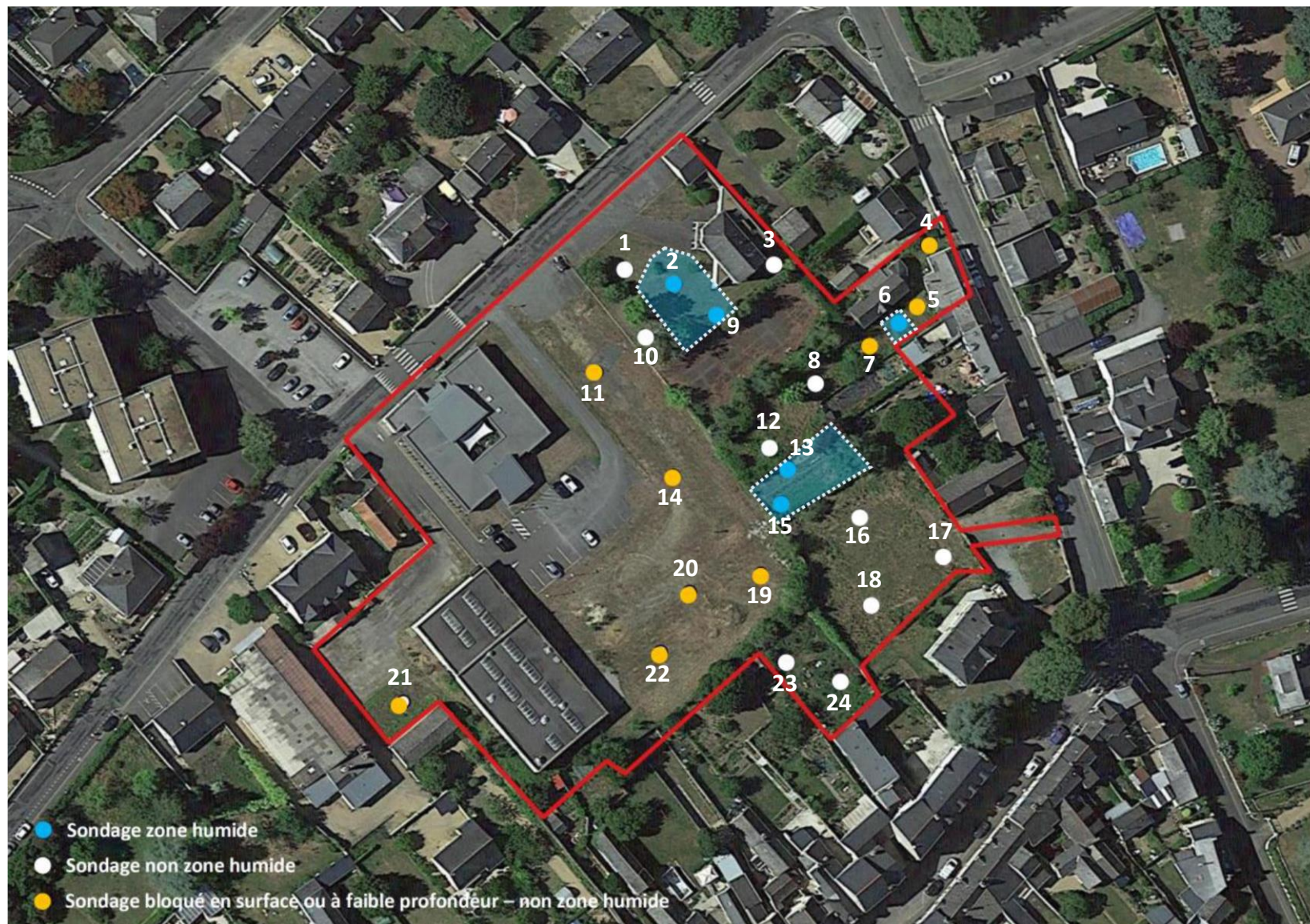
Figure 1 : Localisation des sondages pédologiques et des zones humides
