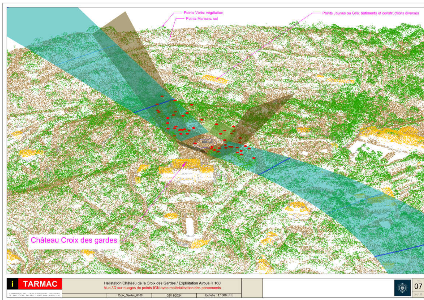
Plots en rouge des percements éventuels à effectuer pour l'hélistation du Château de la Croix des Gardes
