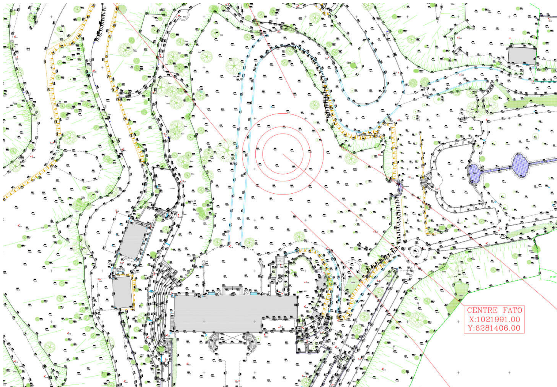
Délimitation du projet de la nouvelle FATO (aire d'approche finale et de décollage)
