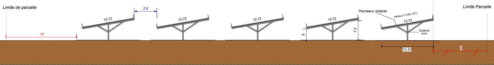
Coupe A-A
